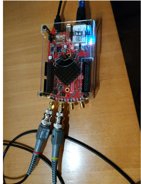
L'oscilloscope utilisé est basé sur un FPGA et une carte « Red Pitaya ».
