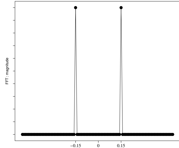
FFT
